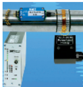
High-Speed Telemetrie mit 50 kHz Bandbreite.
