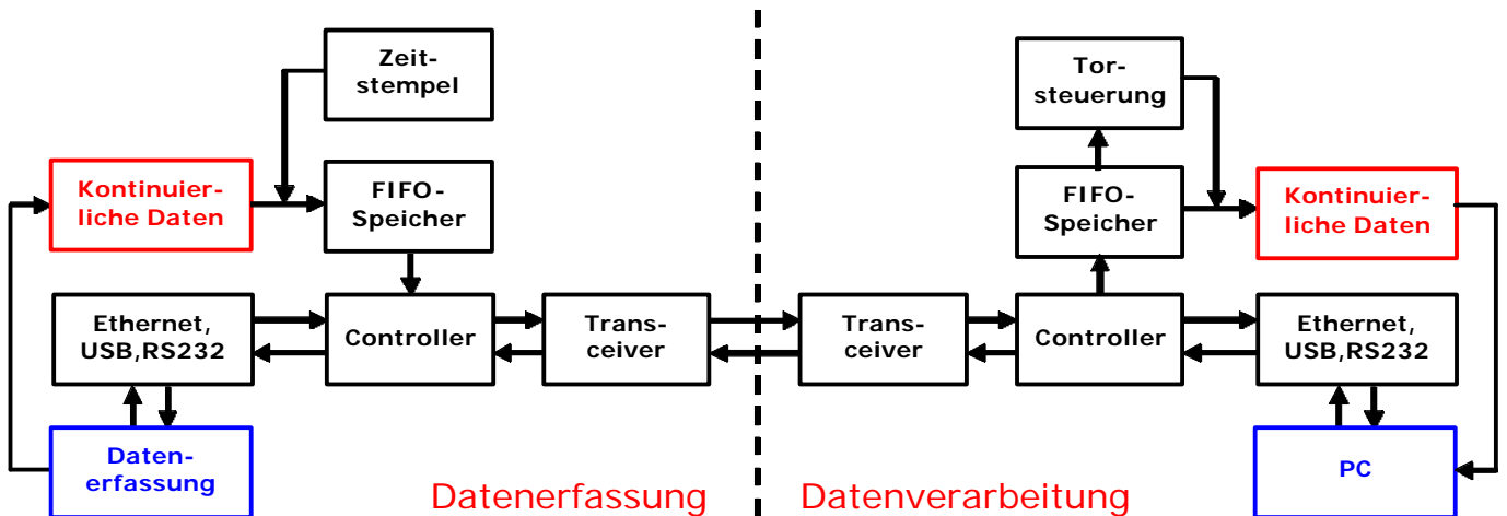
Abb. 2: Blockschaftbild einer bidirektionalen Telemetrieübertragung
