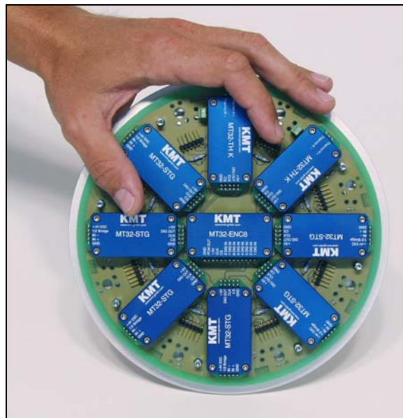
MT32-Disk 8-Kanal-Scheibentelemetrie
