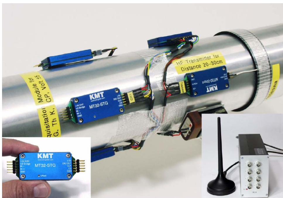
CT8 8-Kanal-Telemetrie mit MT32-Modulen
